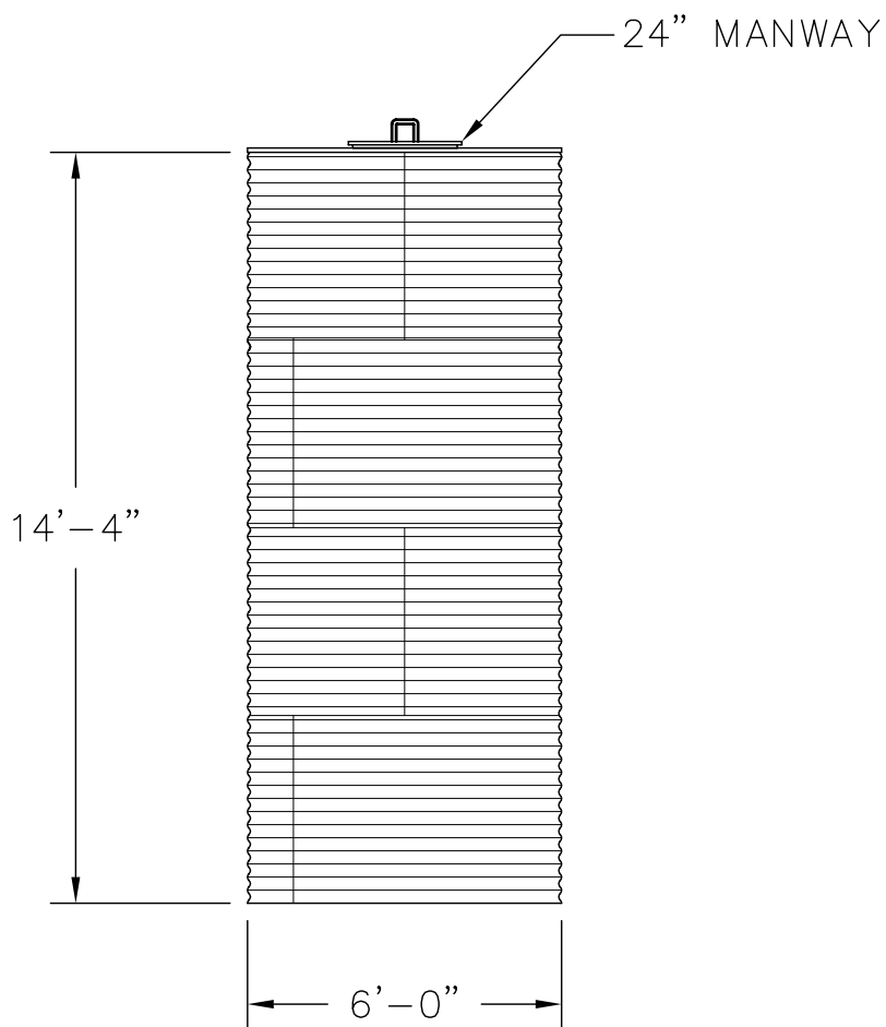
ELEVATION
