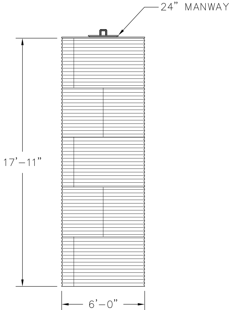
ELEVATION
