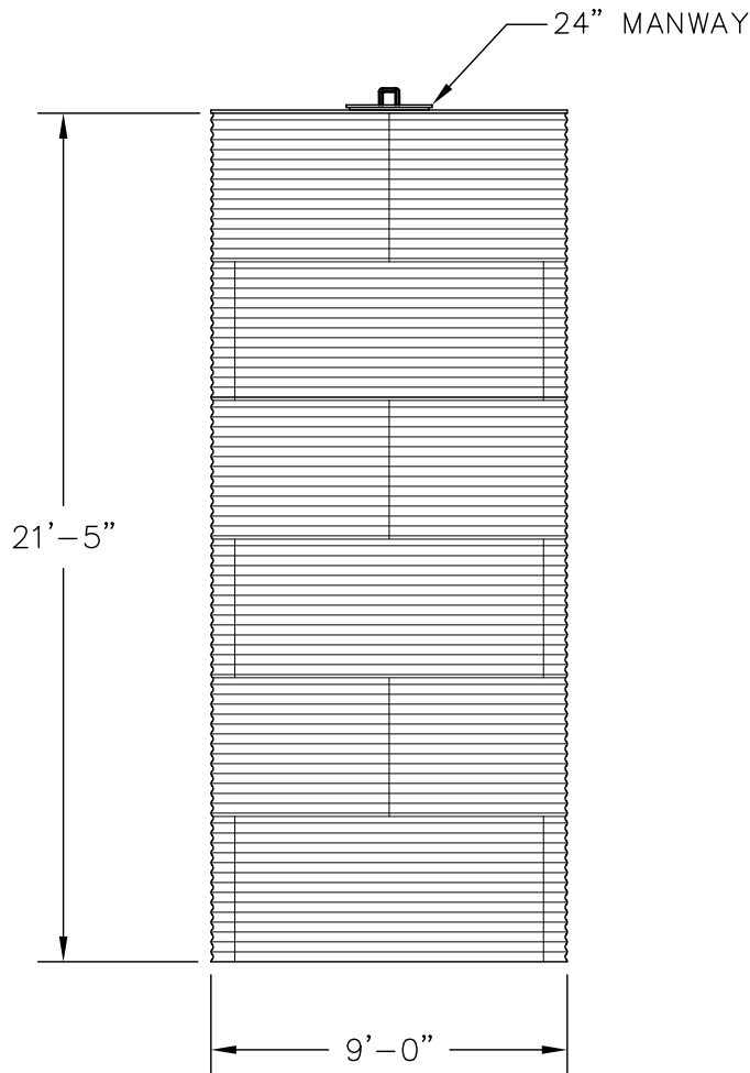
ELEVATION
