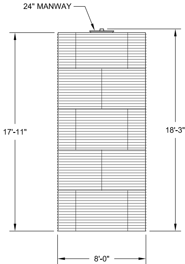
ELEVATION
