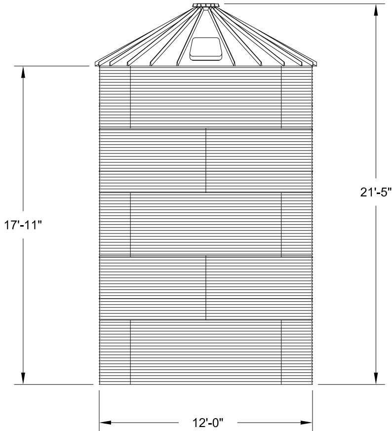
ELEVATION
