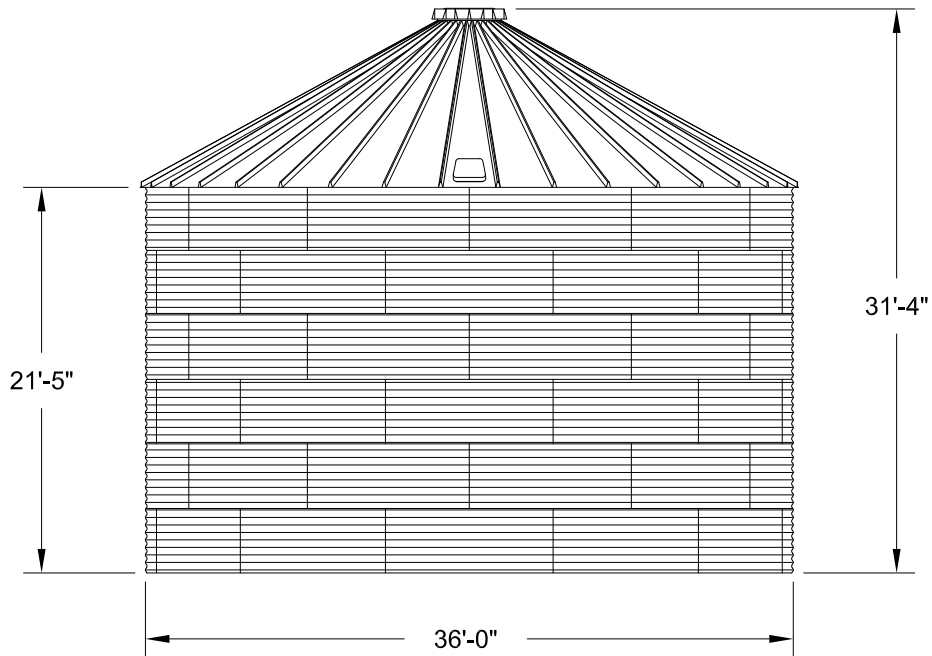
ELEVATION
