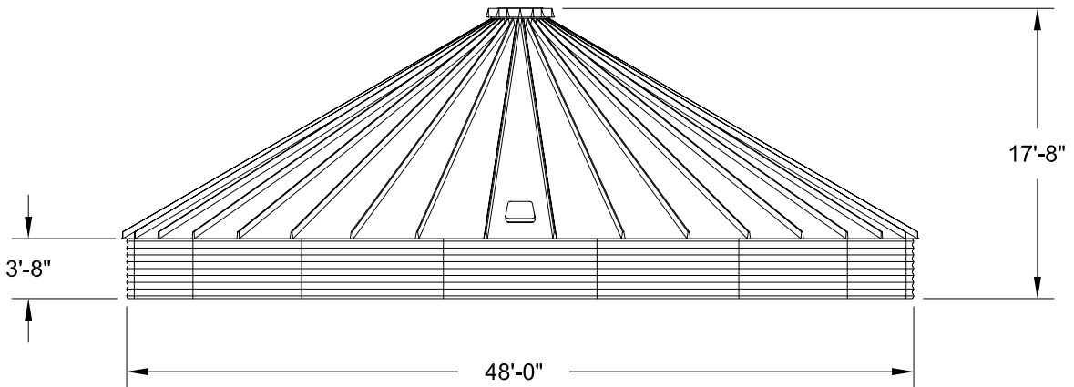
ELEVATION
