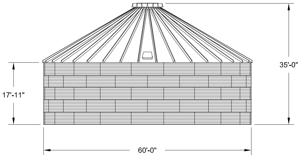
ELEVATION
